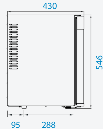
Ansicht von der Seite
