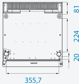
Ansicht von unten
