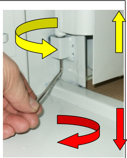
Unteres Türband (Bild 3)
