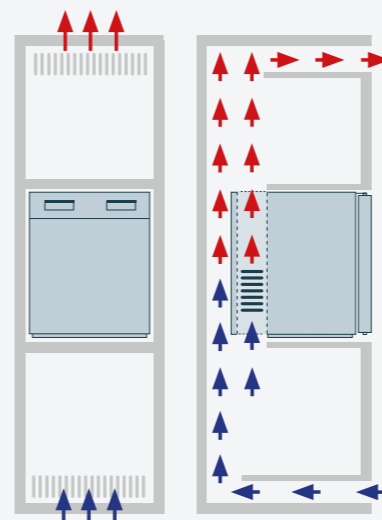
B: Lufteinlass unter und Auslass über einem Fach, freie Zirkulation entlang der gesamten Rückwand
