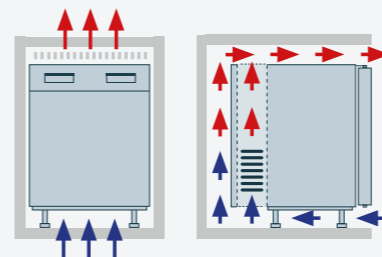
D: Lufteinlass unter und Auslass direkt über der Minibar
