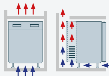
C: Lufteinlass unter der Minibar und Auslass über Lüftungsschlitze oberhalb
